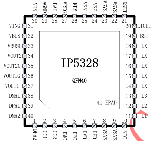
图 2 IP5328 引脚图
