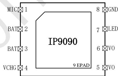
图 2 IP9090 引脚示意图
