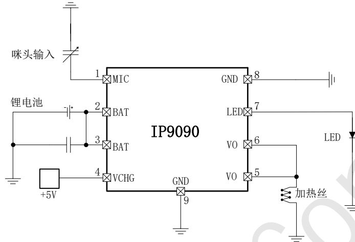
图 4 典型应用原理图
