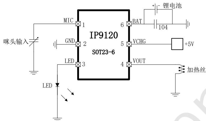
图 4 典型应用原理图
