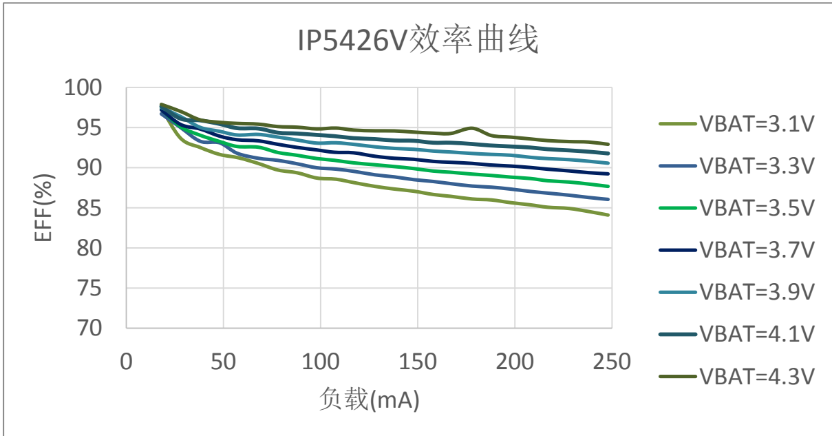
图 4 IP5426V 升压效率图
