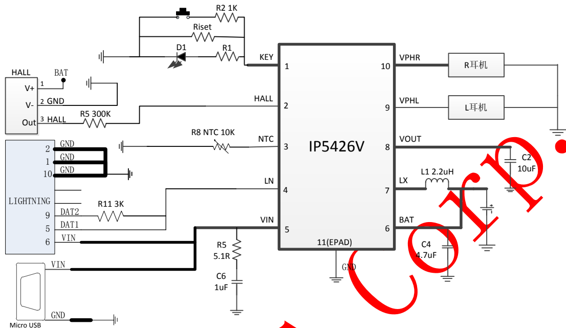
图 18 IP5426V 1LED 灯典型应用原理图
