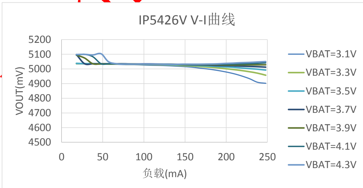
图 5 IP5426V V-I 曲线图
