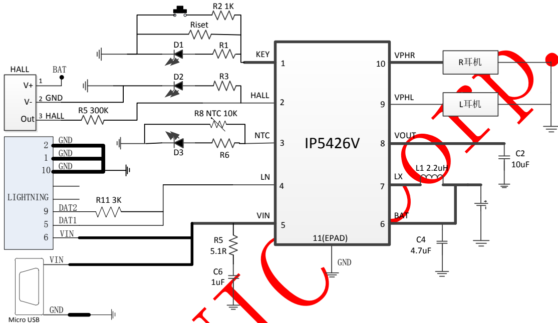
图 16 IP5426V 3LED 典型应用原理图
