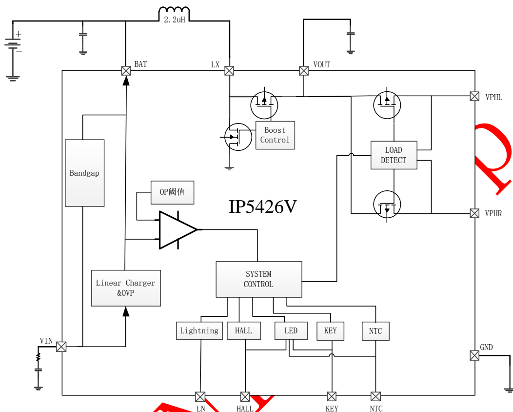
图 3 IP5426V 内部系统框图
