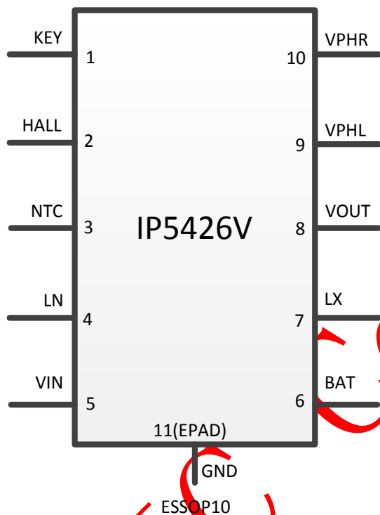
图2 IP5426V 引脚图
