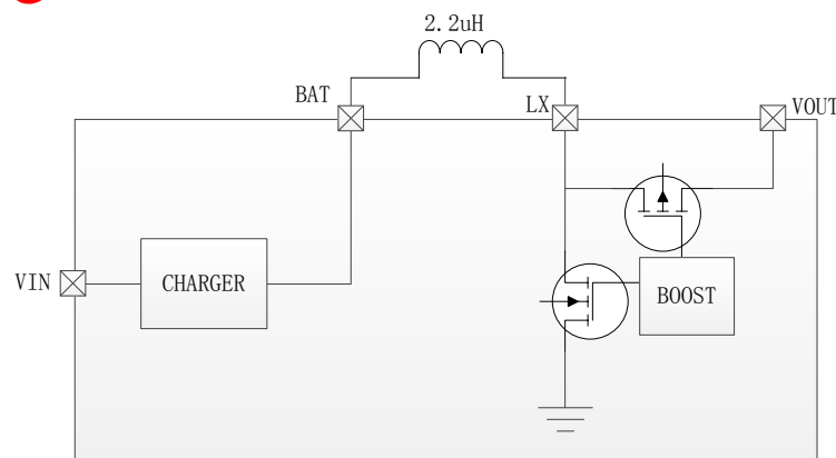
图 7 IP5426V 路径管理示意图
